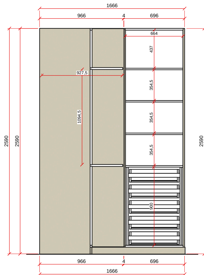
VISTA E - ESC. 1:25
