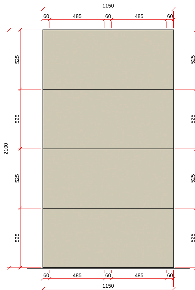
VISTA C - ESC. 1:20
