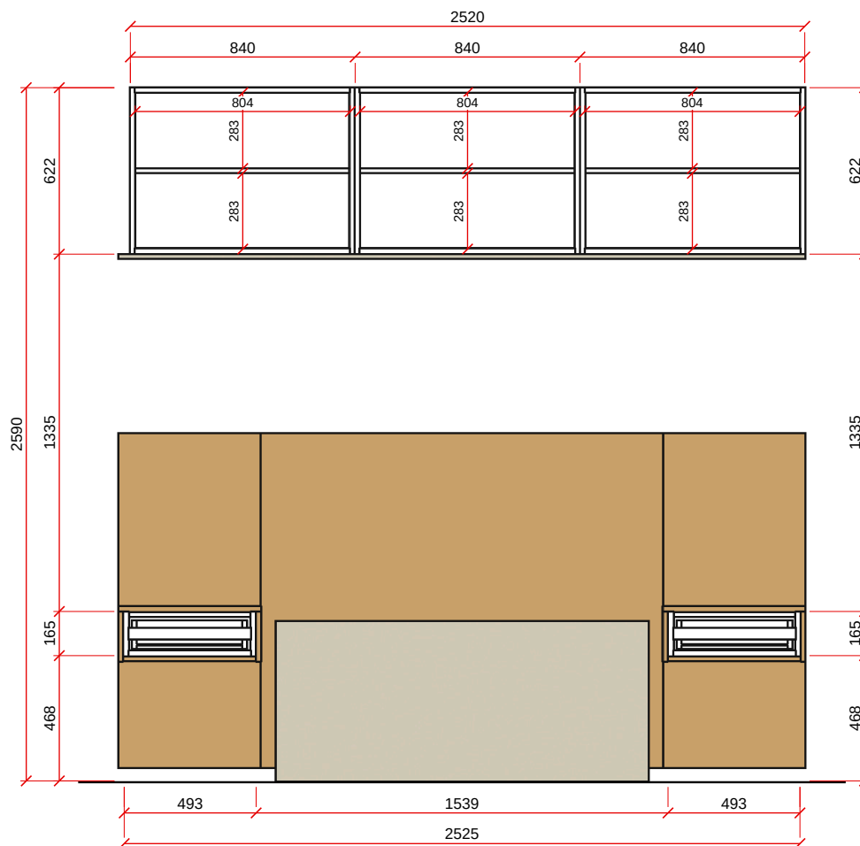
VISTA A - ESC. 1:25
